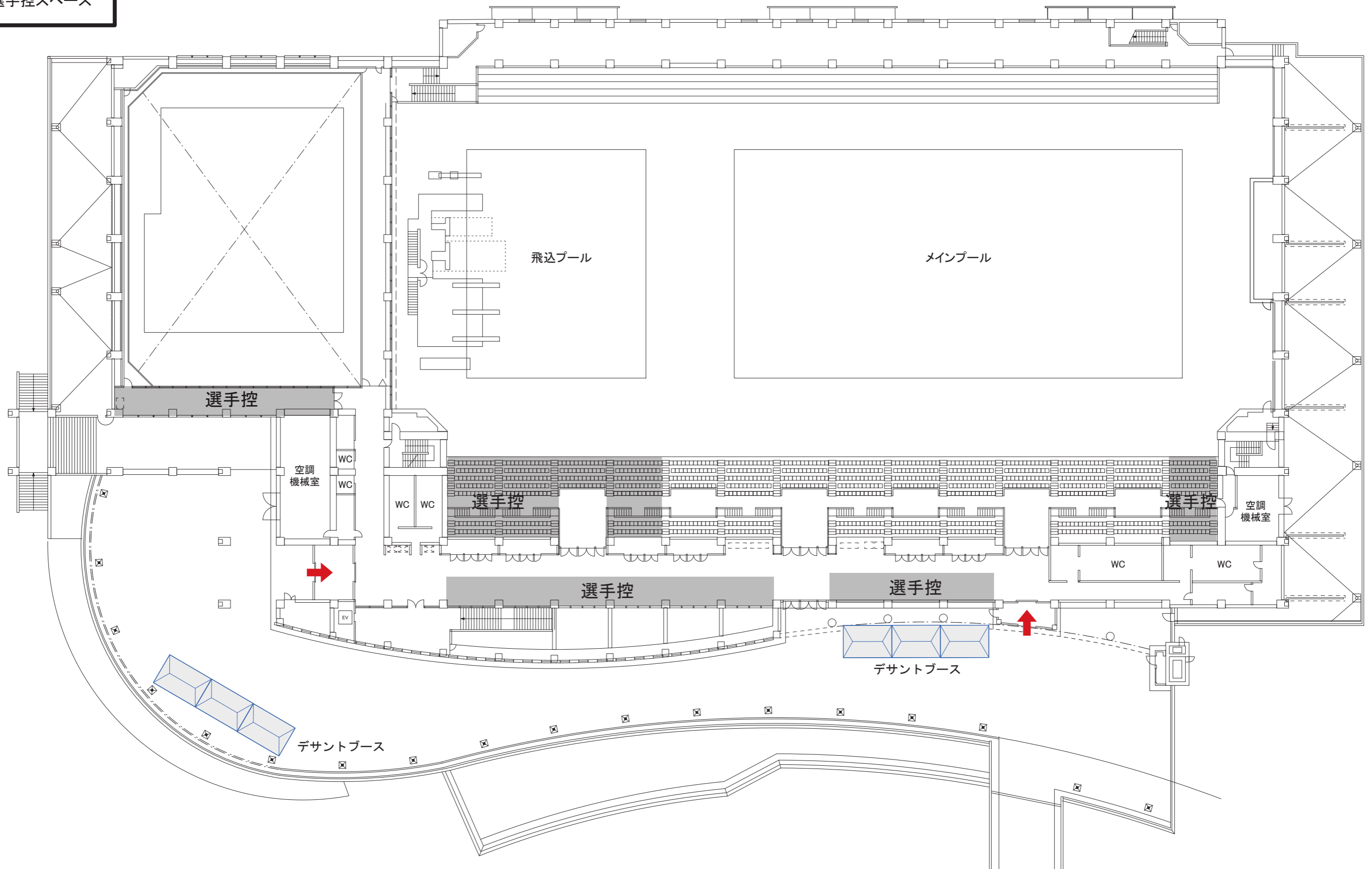
第35回全国JOCジュニアオリンピックカップ春季水泳競技大会 ダイエープロビスフェニックスプール2階平面図
